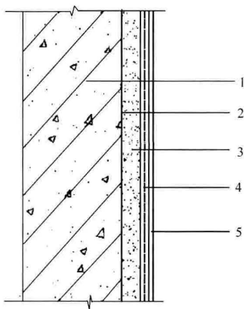
图 A.0.3 无机轻集料砂浆内保温系统基本构造示意 1—混凝土墙及各种砌体墙基层；2—界面砂浆，基层为蒸压加气混凝土时采用专用界面砂浆；3—无机轻集料保温砂浆保温层； 4—抗裂砂浆及耐碱玻纤网布；5—涂料饰面作饰面层
