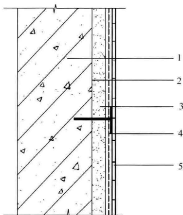
图 A.0.2 面砖饰面无机轻集料砂浆外墙外保温系统基本构造示意 1—混凝土墙及各种砌体墙基层；2—界面砂浆，基层为蒸压加气混凝土时采用专用界面砂浆；3—无机轻集料保温砂浆保温层；4—抗裂砂浆及耐碱玻纤网布，有加强要求的可增设一道耐碱玻纤网布，加锚固件； 5—面砖作饰面层
