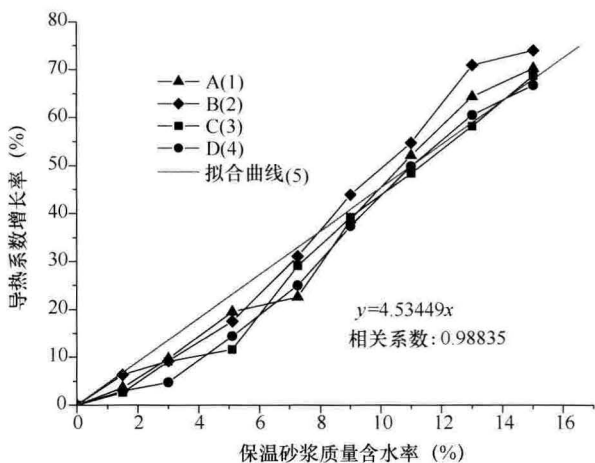
图 1 导热系数随质量含水率变化曲线
