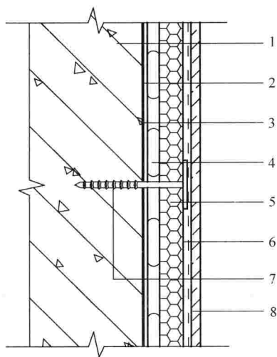
图 5.2.3 复合板薄抹灰保温系统基本构造
