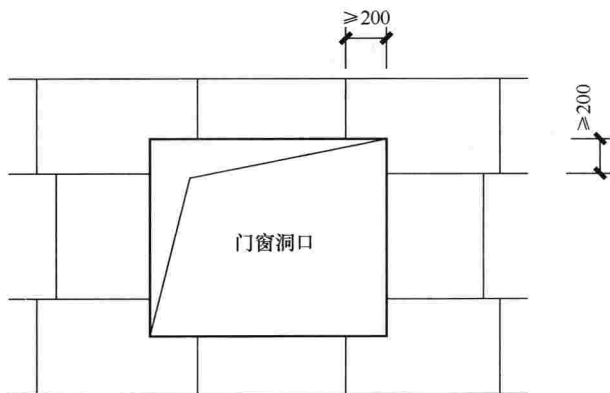
图 6.2.4-2 门窗洞口处复合板排列图
