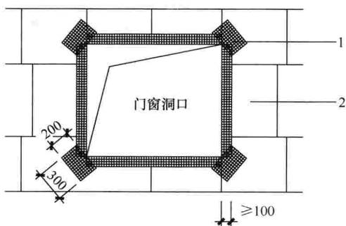
图 5.2.8 门窗洞口部位玻纤网增强示意图
