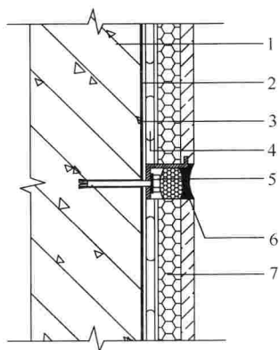
图 5.3.2 有饰面复合板保温系统基本构造
