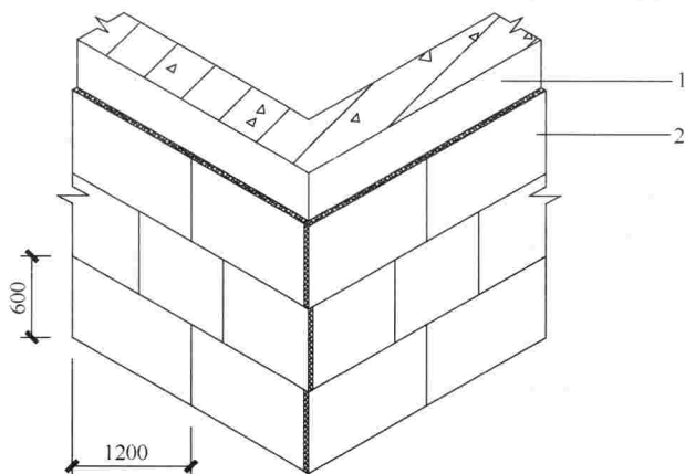
图 6.2.4-1 墙角处复合板排板图
